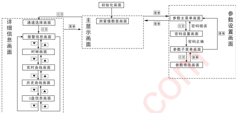
图 5.3 运行和操作流程图
