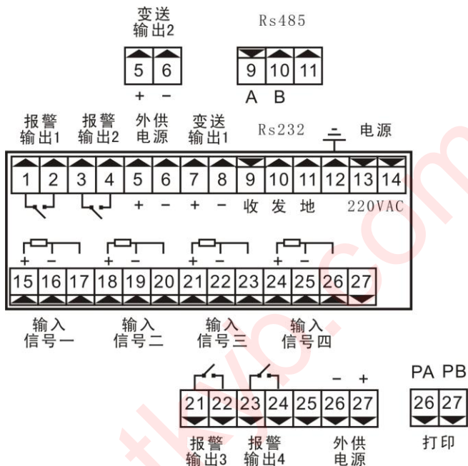
图 4.3 仪表接线端子图
